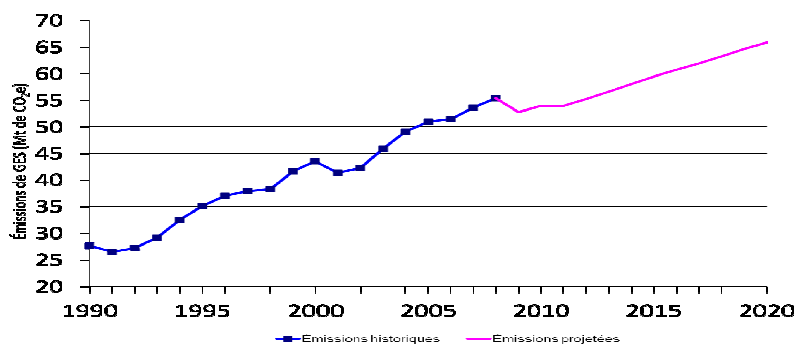
Figure EN17: Tendance des émissions des gaz à effet de serre (GES) des véhicules moyens et lourds (1990-2020)
