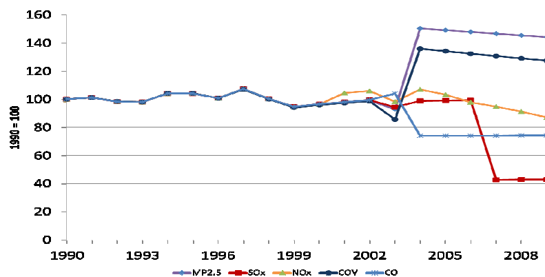
Figure EN14: Tendances des émissions de polluants atmosphériques du transport ferroviaire (marchandises et passagers) (1990-2009)
