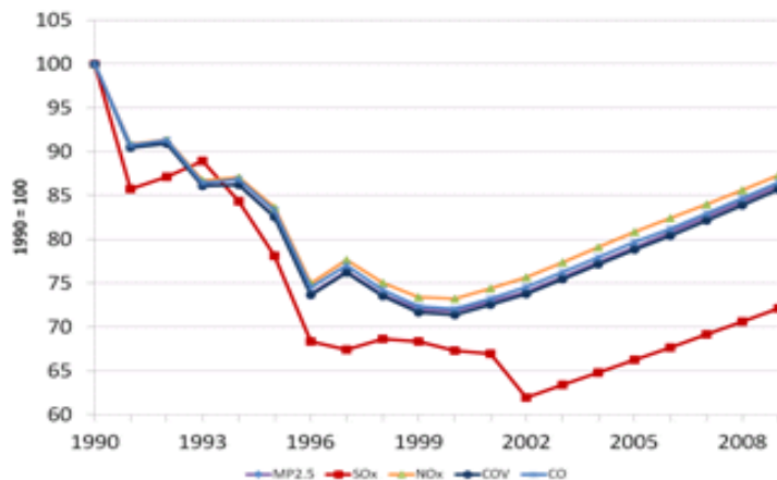
Figure EN11: Tendances des émissions de polluants atmosphériques du transport maritime (1990-2009)
