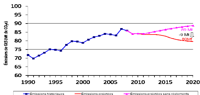
Figure EN15: Tendance des émissions des gaz à effet de serre (GES) des véhicules légers (1990-2020)
